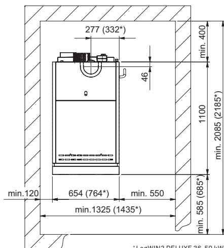
Draufsicht
